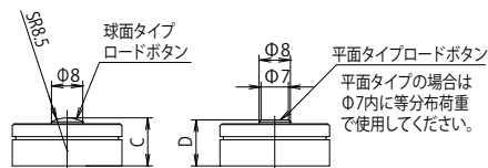
球面タイプ 平面タイプ
