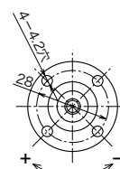
(矢印はφ6中心軸に対する負荷方向)
