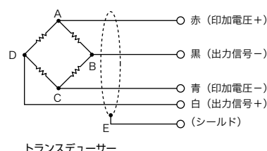
ケーブルおよびコネクタ結線図
