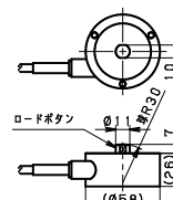
ロードボタン取付寸法図
