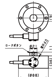
ロードボタン取付寸法図
