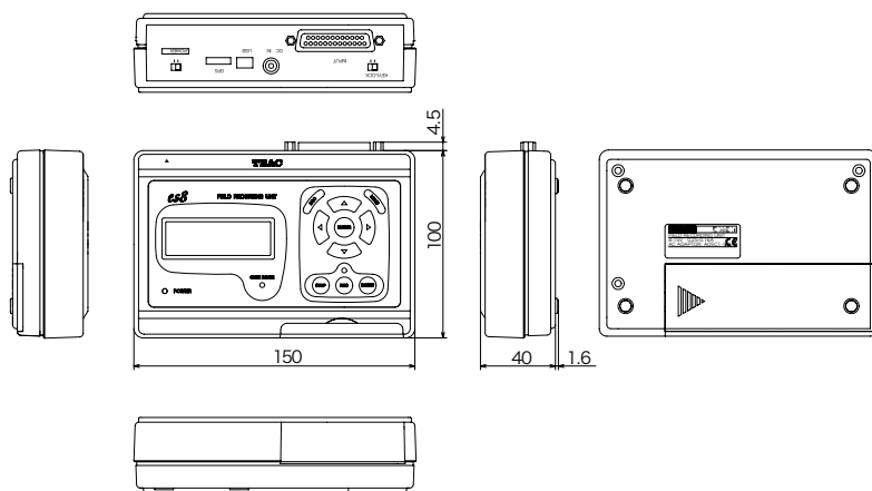
■ 外形寸法図 (単位: mm)
