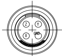
[矢視(A)図]
